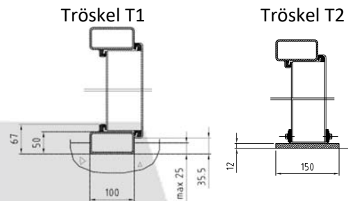
Exempel på tröskel T1 och T2 vid karmdjup 100mm
